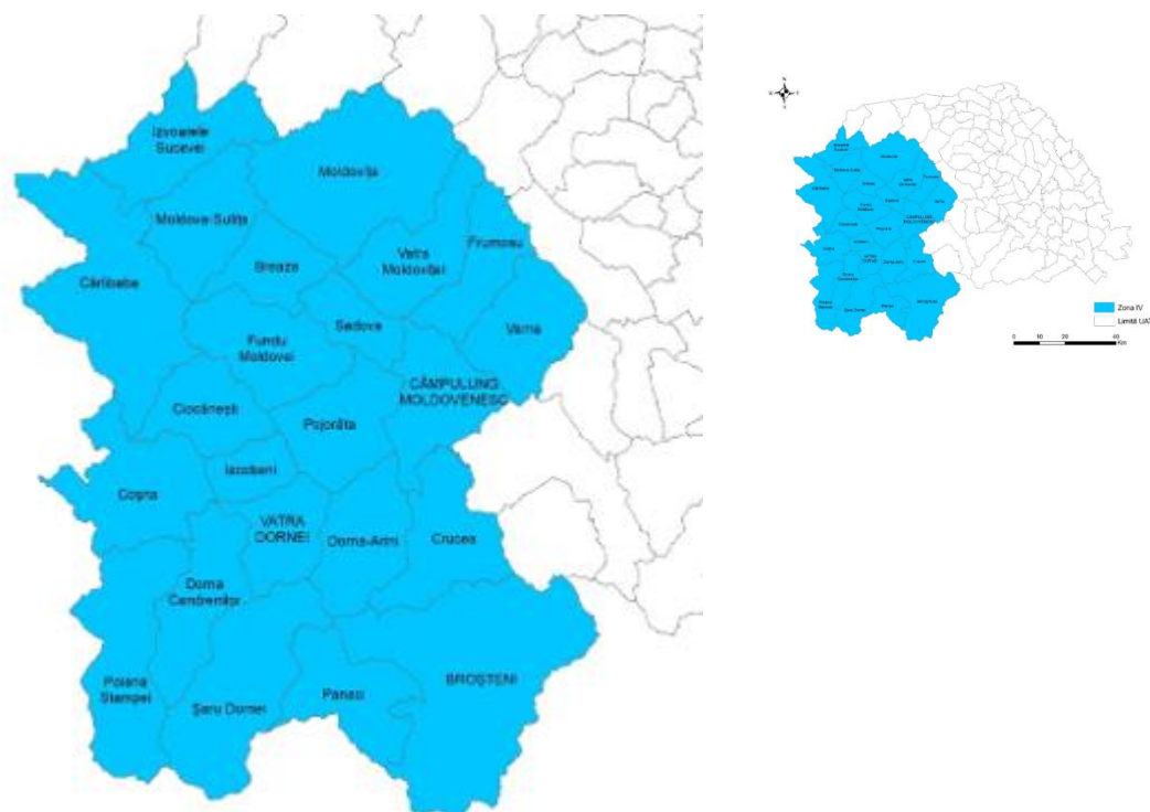
Figura 1 – Aria delegată
